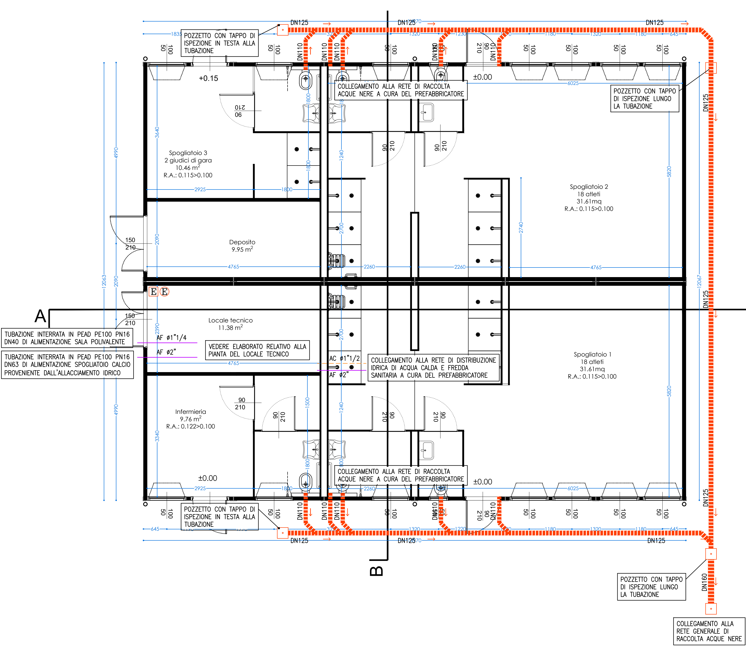
SPOGLIATOIO CALCIO – IMPIANTO IDRICO SANITARIO E SCARICO ACQUE NERE SCALA 1:50
