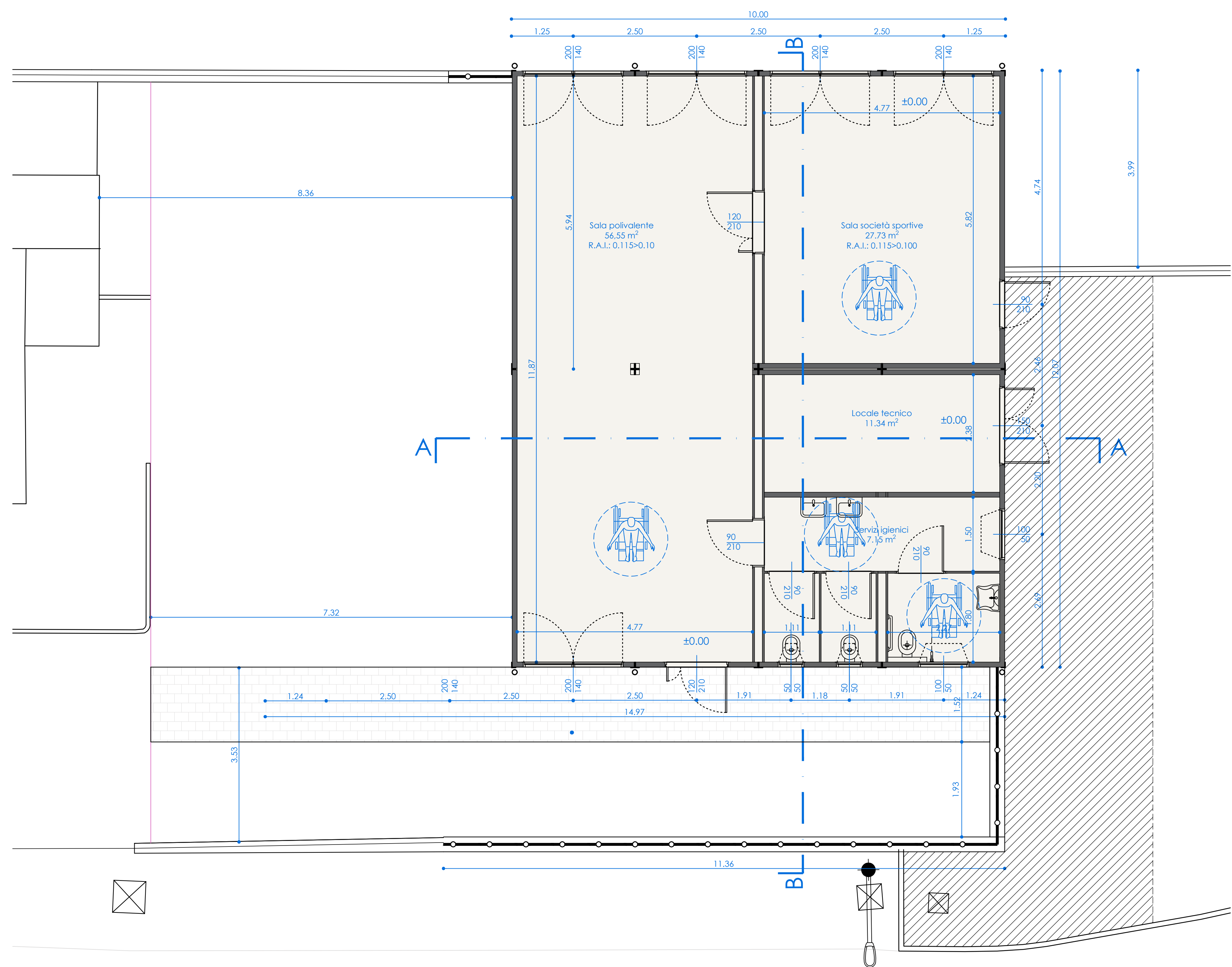
PIANTA BLOCCO SALA POLIVALENTE/BAR scala 1:50
