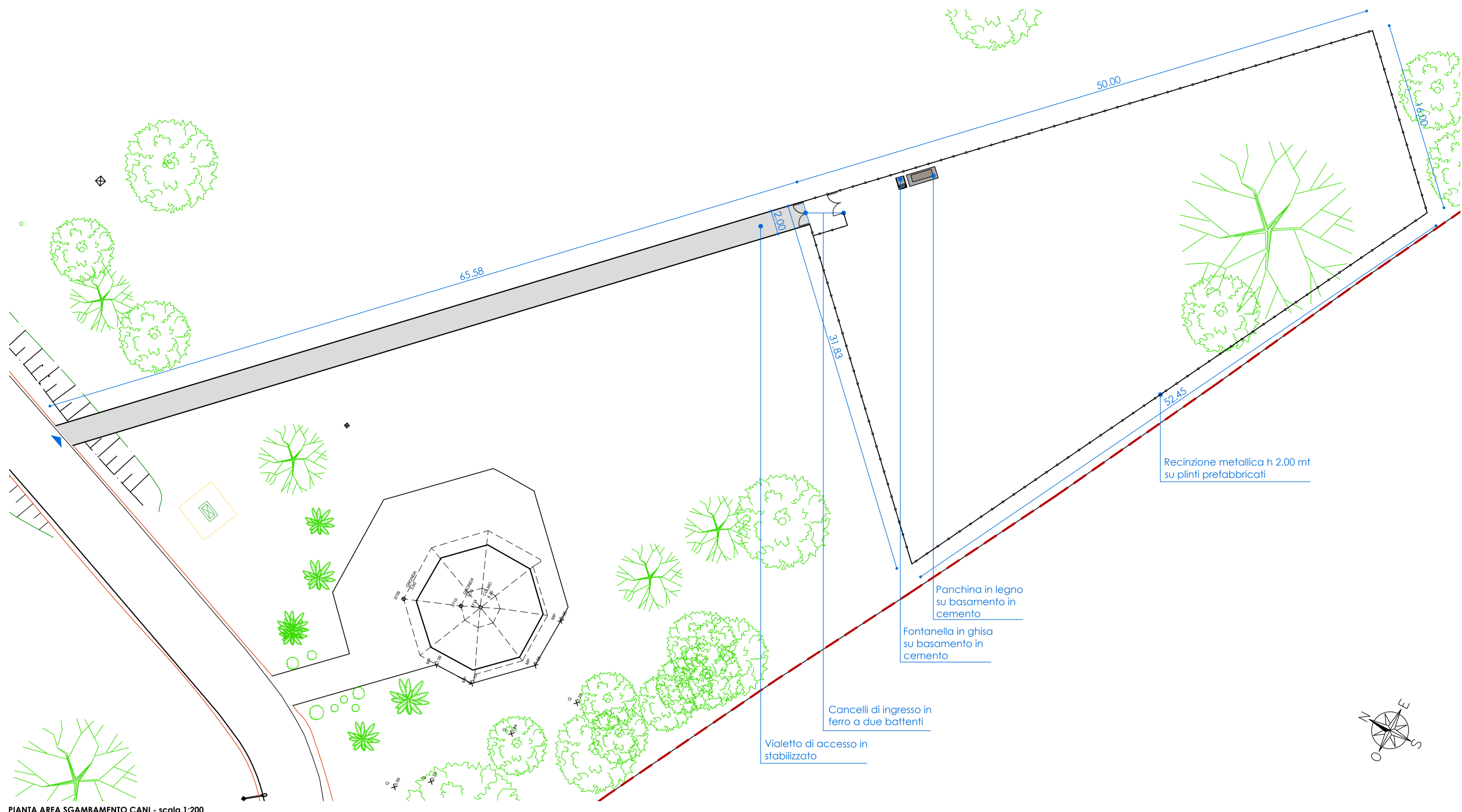
PIANTA AREA SGAMBAMENTO CANI - scala 1:200
