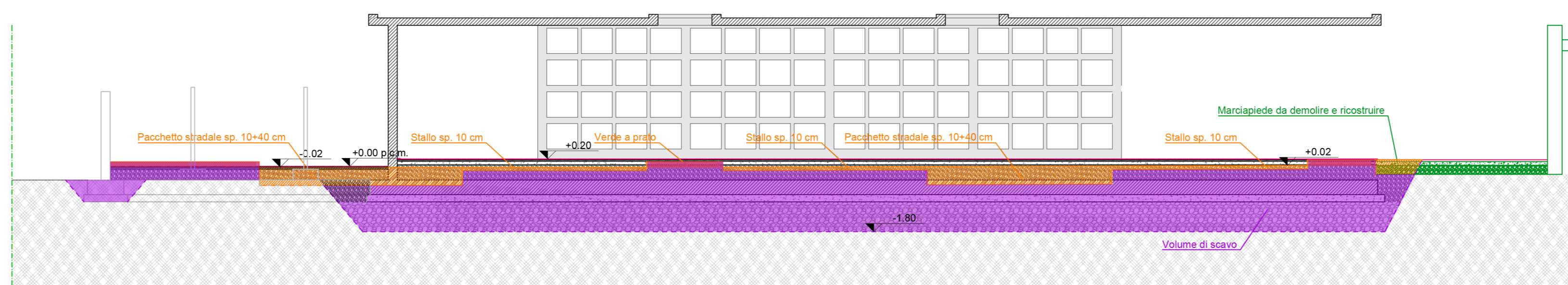
SEZIONE AA - Sovrapposto stato attuale stato di progetto Scala 1:100
