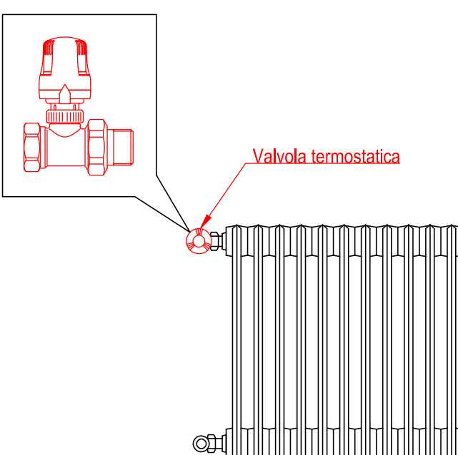
Particolare installazione valvole termostatiche STATO DI PROGETTO
