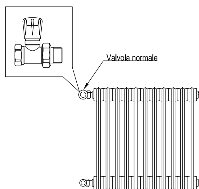
Particolare installazione valvole termostatiche STATO DI FATTO
